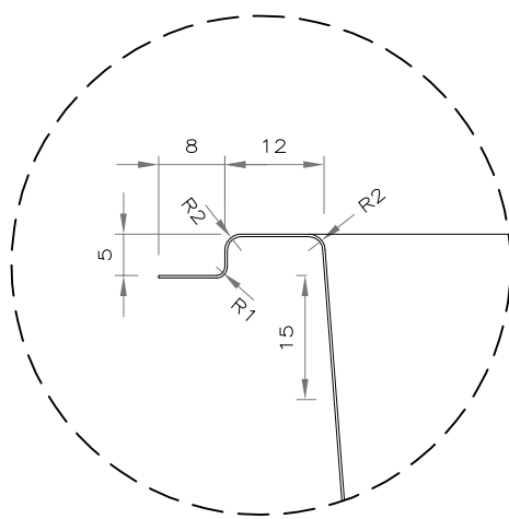
Detalhe 3 Escala 1/10
