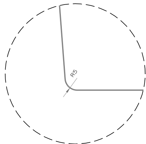
Detalhe 4 Escala 1/10
